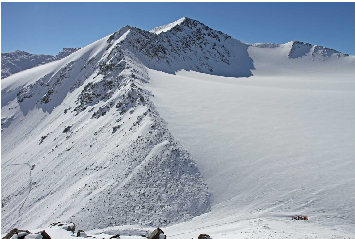
Рис. 18: Вид с гребня Джаникту на перевал Рубцовский
